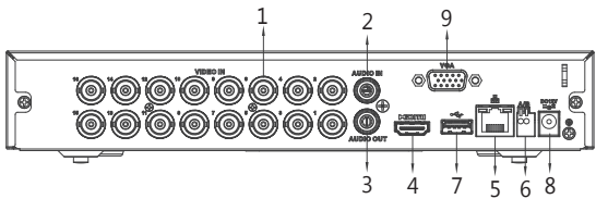
DHI-XVR5116HS-S2
